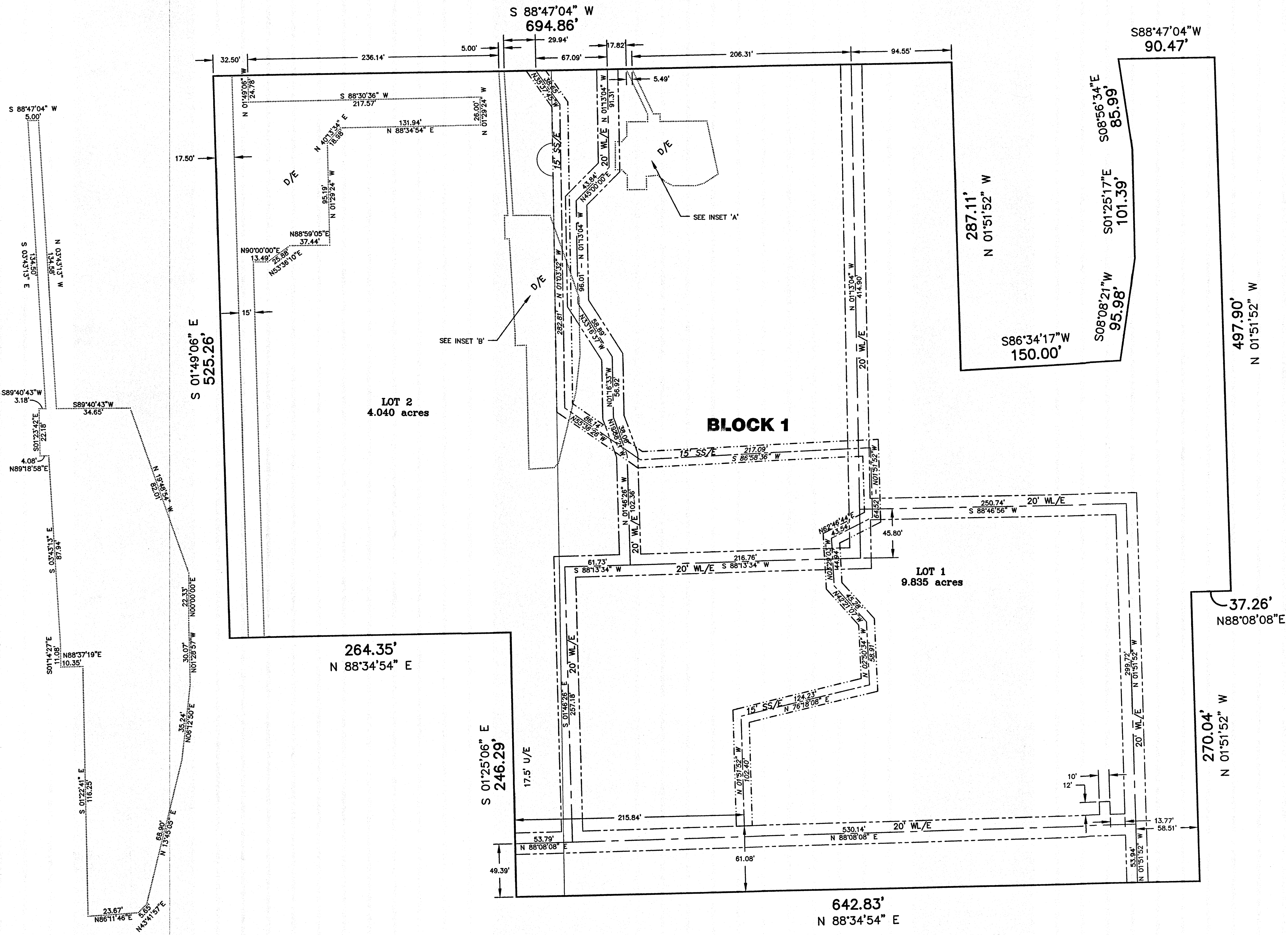
INSET 'B'
