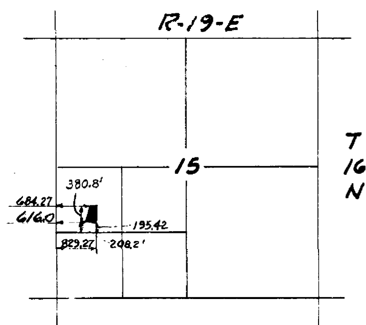
SECTION PLAT
